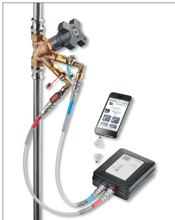
Système de mesure «OV-DMC 3» réf. 1069278 avec « Hydrocontrol VTR »
