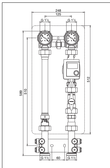
Illustr. 4.2 Dimensioni del gruppo di collegamento al circuito di riscaldamento
