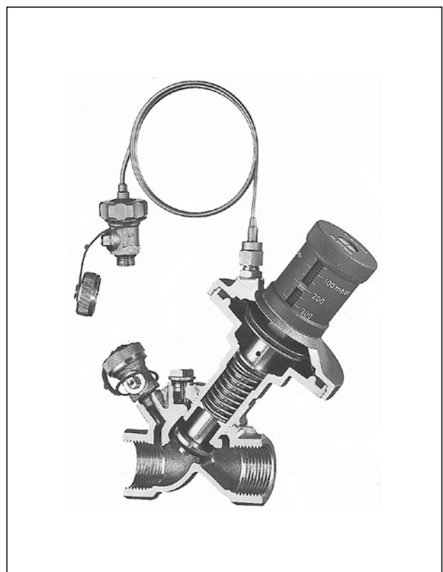
Przekrój
