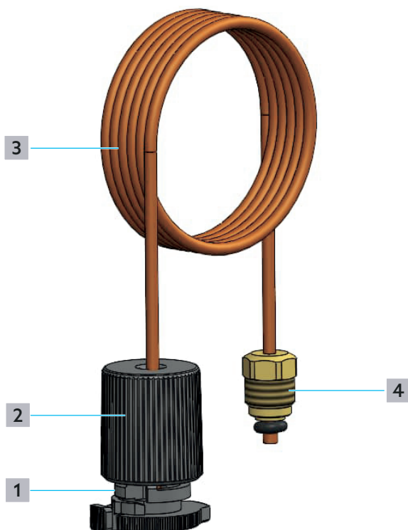
Abb. 6: Aufbau Impulsleitung
