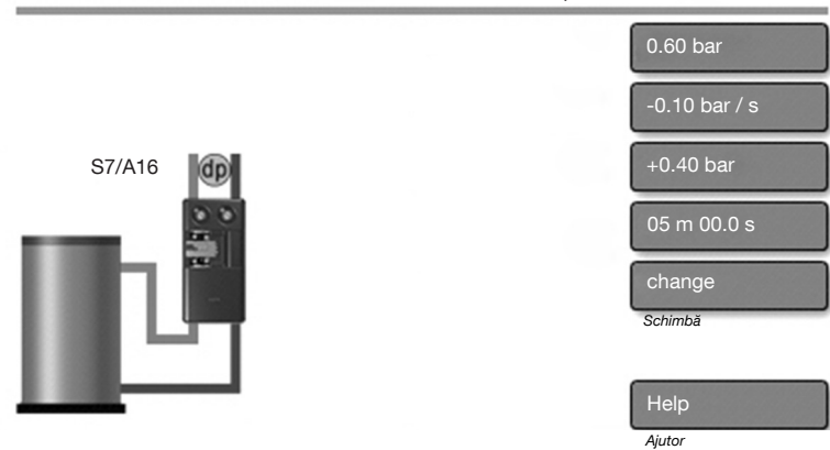
Reglarea presiunii diferențiale pe coloană Differential pressure control in the riser
