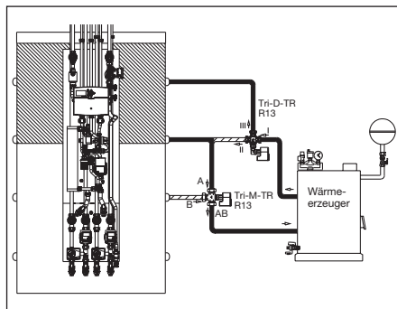
Abb. 5.1 Beladung Hochtemperaturbereich
