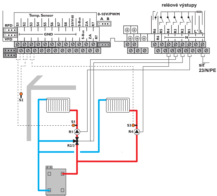
Schéma 6: smíšený a nesmíšený topný okruh
