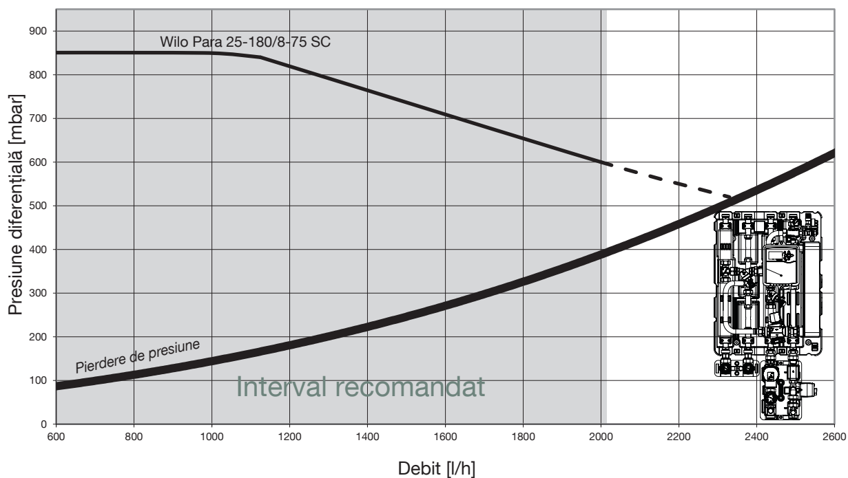
Fig. 5: Pierdere de presiune circuit secundar Regudis H-HT
