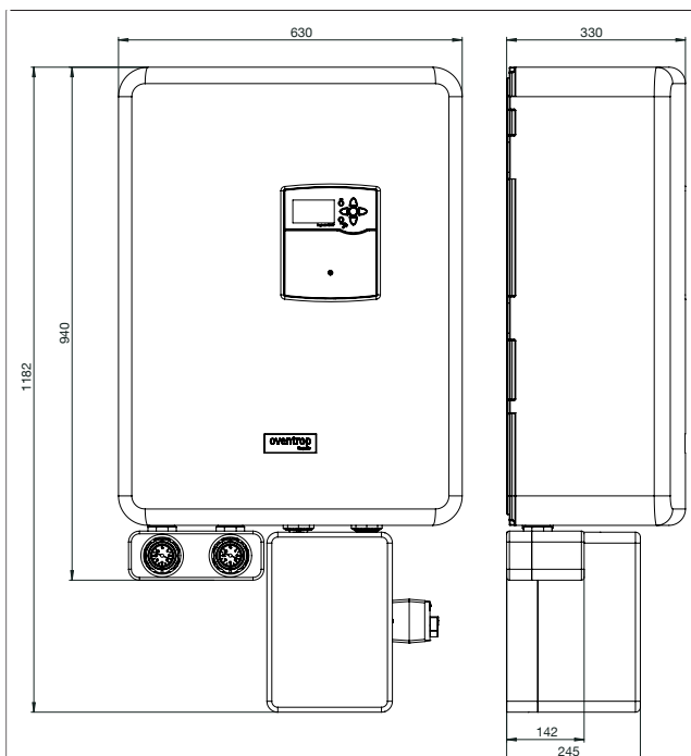
Fig. 3: Dimensiuni în mm
