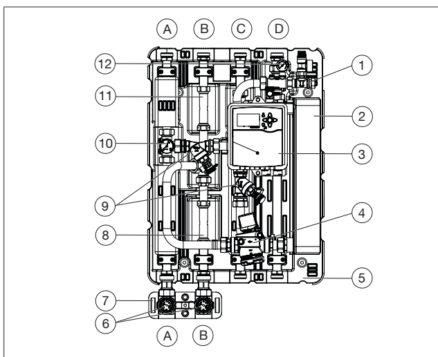
Fig. 2: Structură Regudis H
