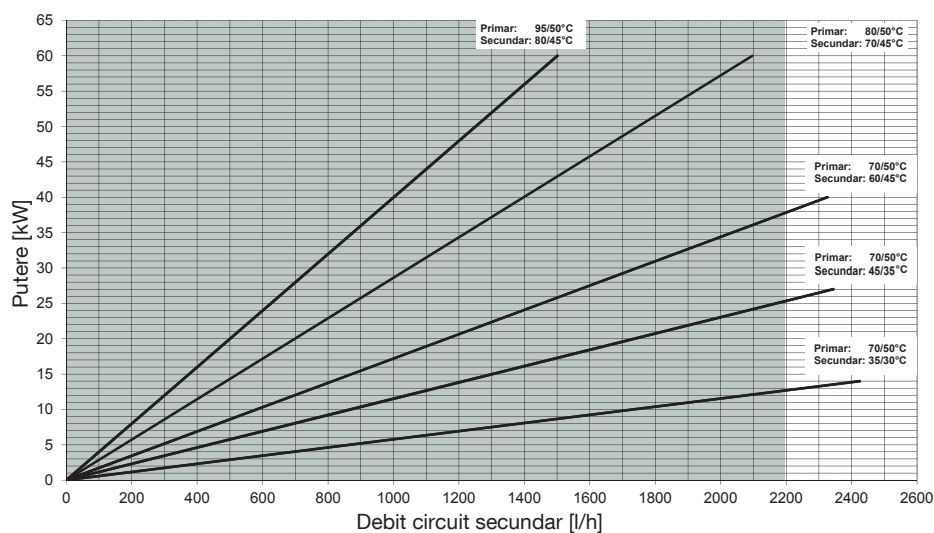
Fig. 8: Diagramă de performanță; debitul max. recomandat al Regudis H în combinație cu Regumat M 3
