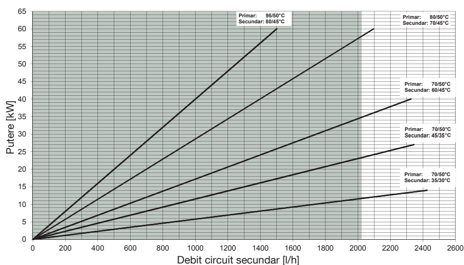
Fig. 6: Diagramă de performanță; debitul max. recomandat al Regudis H în combinație cu modulul de comutare
