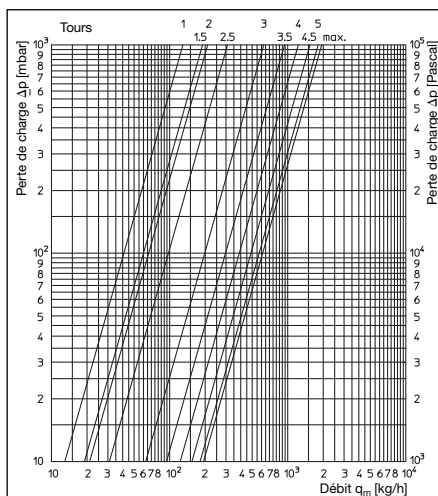
Fig. 9.1: Diagramme mécanique de réglage pour différents prérégles, mécanisme ouvert
