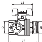
Рис. 4.2. Длина гребенки из нержавеющей стали „Multidis SF“
