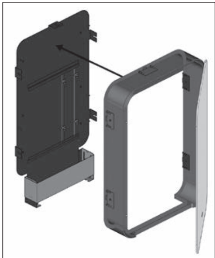
Abb. 4.1 Montage „Regubox“ Exklusiv-Verteilerschrank
