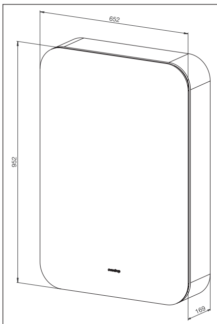
Abb. 3.1 Abmessungen
