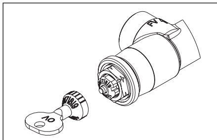
Abb. 10 Voreinstellung Thermostatventil
