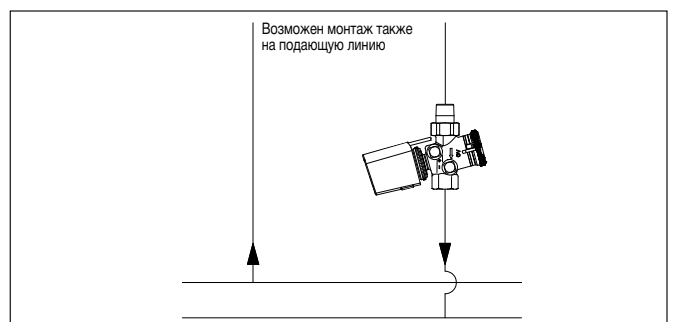
Пример: Регулирования расхода с помощью вентиля „Cocon QTZ“.
