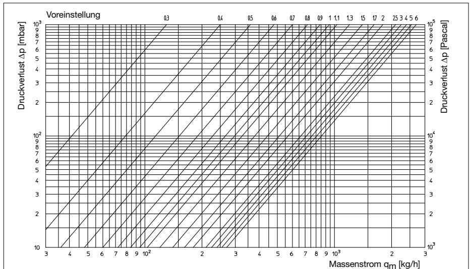
Abb. 9.1: Diagramm „Hycocn VTZ“ Strangregulierventil DN 20
