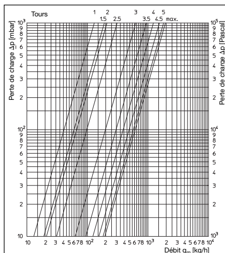
Fig. 9.1: Diagramme mécanique de réglage pour différents préréglages, mécanisme ouvert
