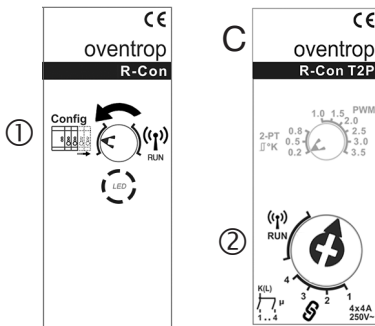
Abbildung 21: Neukonfiguration „R-Con“ nach Einbau Erweiterungsmodul
