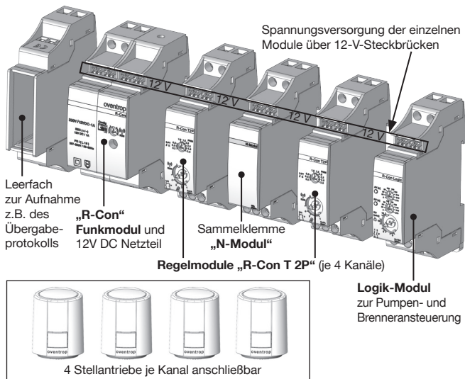
Abbildung 6: Übersicht Bedienelemente und Schraubklemmen am „R-Con“
