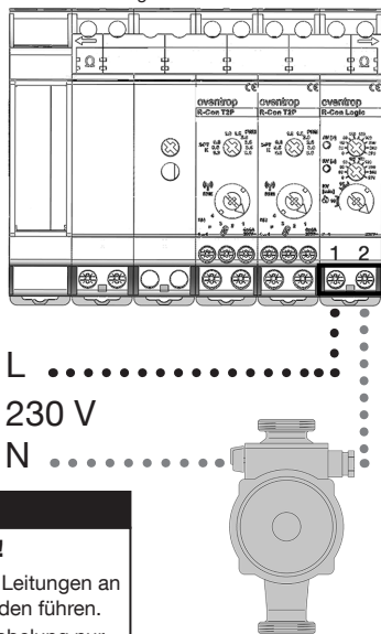
Abbildung 23: Verkabelung für Pumpenanschluss an Logik-Modul
