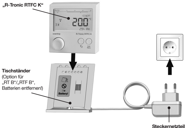
Abbildung 10: Montage „R-Tronic“ auf Tischständer
