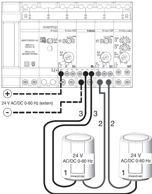
Abbildung 17: Anschluss Stellantriebe an 24 Volt über Regelmodul
