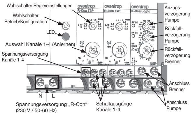
Abbildung 6: Übersicht Bedienelemente und Schraubklemmen am „R-Con“
