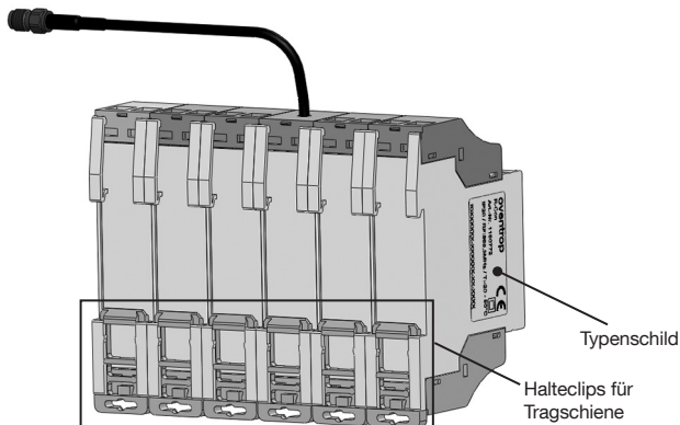
Abbildung 4: Rückansicht des Funkempfängers „R-Con“
