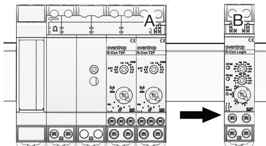
Abbildung 19: Ablösung Logik-Modul von Funkempfänger
