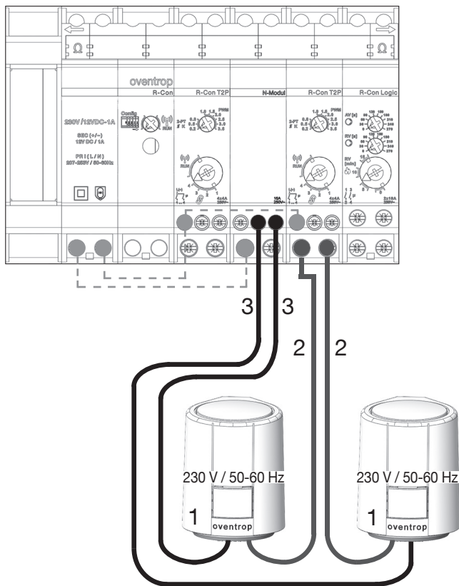
Abbildung 16: Anschluss Stellantriebe an 230 Volt über Regelmodul
