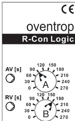
Abbildung 42: Einstellung Anzugs- und Rückfallverzögerung Pumpenlogik
