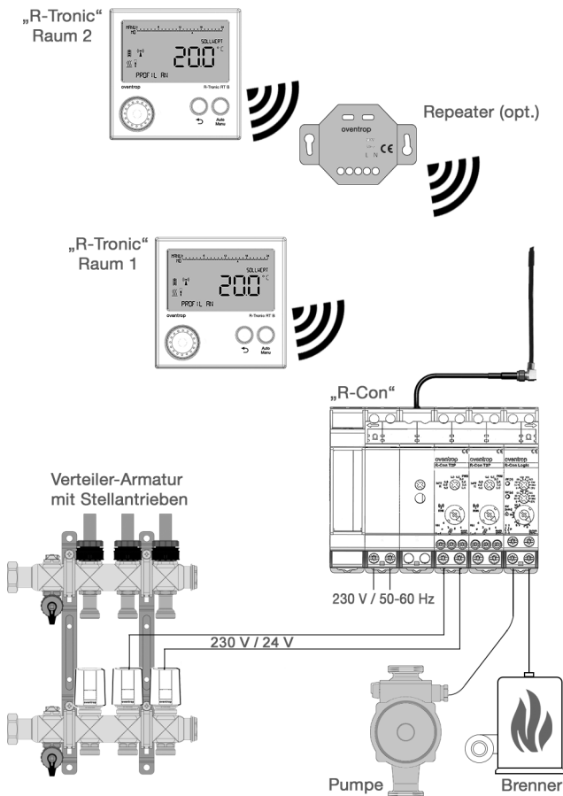
Abbildung 1: Einsatz Funkempfänger mit „R-Tronics“ und Heizungsanlage (Beispiel)
