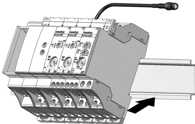
Abbildung 12: Fixierung des Funkempfängers an Tragschiene
