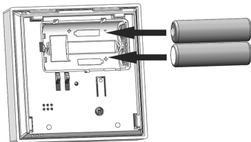
Abbildung 7: Batterieeinsatz „R-Tronic“
