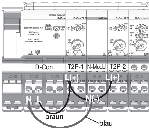
Abbildung 15: Mitgelieferte Kabelbrücken einsetzen
