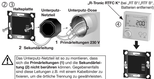
Abbildung 9: Wandmontage Halteplatte „R-Tronic“ mit Unterputznetzteil
