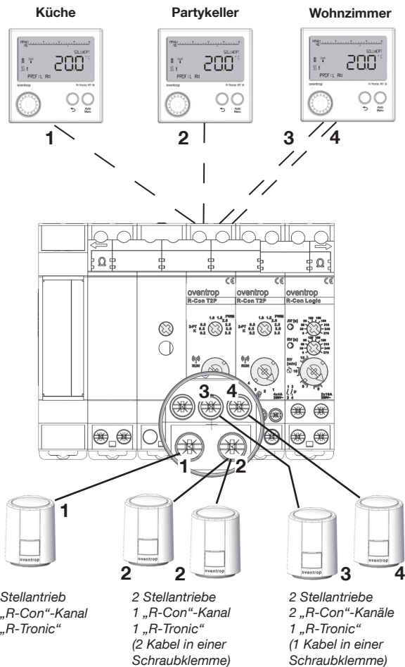
Abbildung 33: Beispielskizze für Kanalzuweisungen an „R-Tronics“
