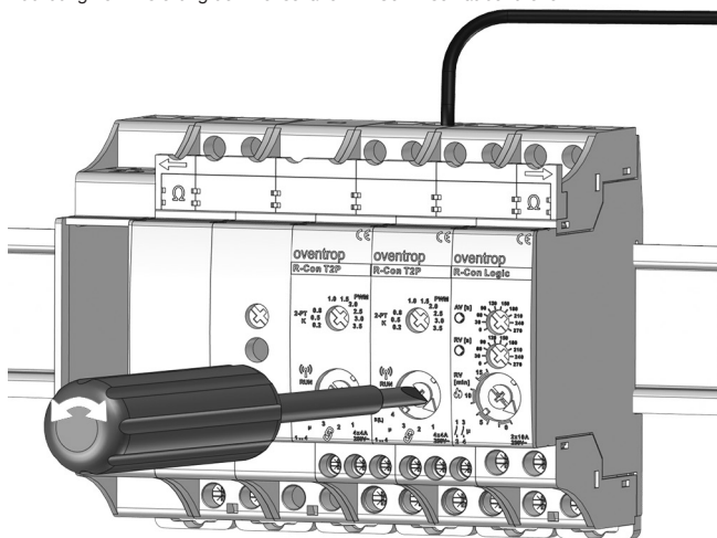
Abbildung 13: Einstellung der Drehschalter mit Schlitzschraubendreher
