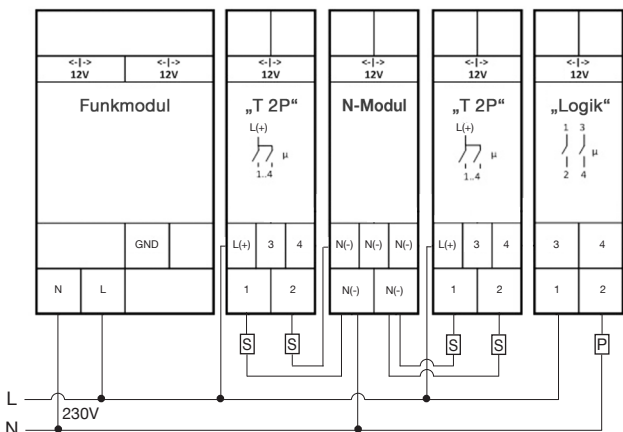
Abbildung 25: Übersicht Anschluss-Schema 230 Volt
