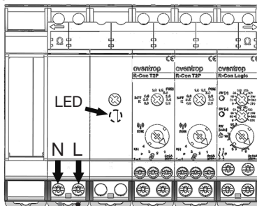
Abbildung 24: Anschluss Funkempfänger an 230-Volt-Netz
