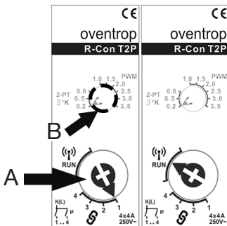
Abbildung 30: Anlernen an „R-Tronic“: Auswahl eines Kanals am Regelmodul
