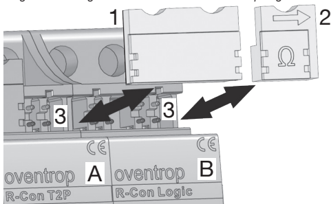
Abbildung 18: Ablösung 12-V-Steckbrücken von Funkempfänger
