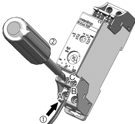
Abbildung 14: Anschluss von Kabelhülsen an Schraubklemmen Regelmodul
