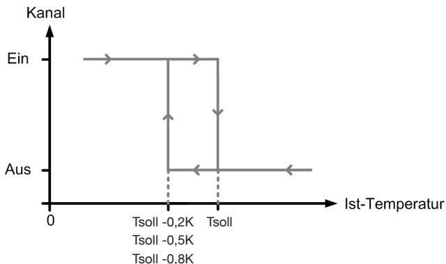
Abbildung 40: Prinzip des 2-Punkt-Verhaltens
