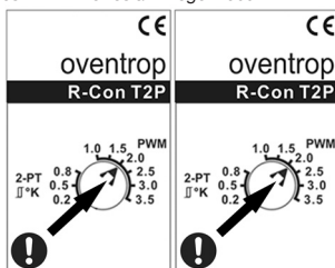
Abbildung 39: Einstellen des PWM-Wertes am Regelmodul
