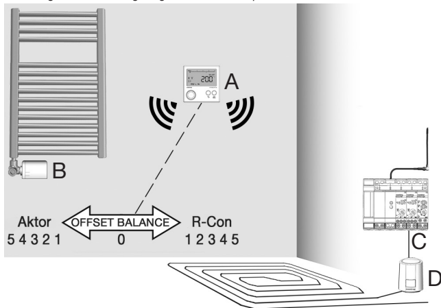
Abbildung 62: Balance-Regelung zwischen Heizkörper und Flächenheizkreis
