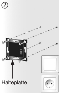
Abbildung 8: Wandmontage Halteplatte (Batteriebetrieb)
