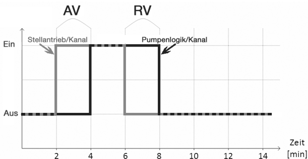
Abbildung 41: Diagramm Anzugs- und Rückfallverzögerung der Pumpenlogik
