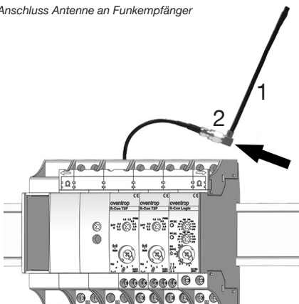
Abbildung 27: Anschluss Antenne an Funkempfänger
