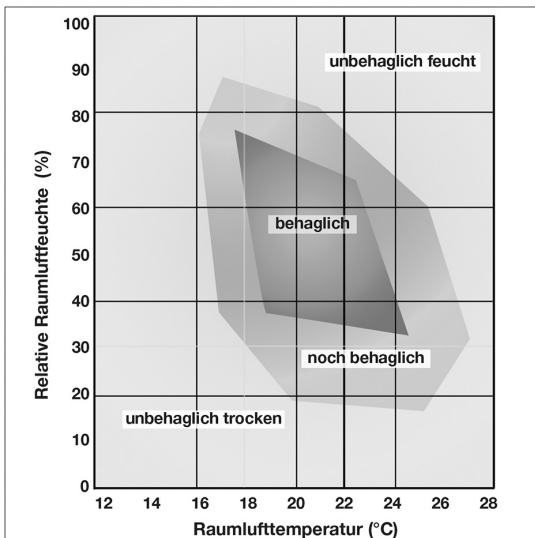
Abbildung 69: „Behaglichkeitsdiagramm“
