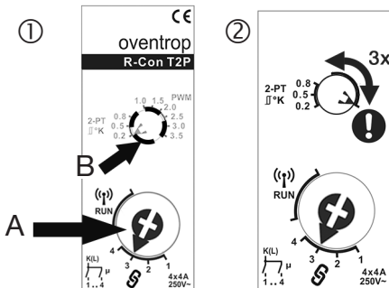
Abbildung 35: Einzelne Kanäle für Funkthermostate löschen
