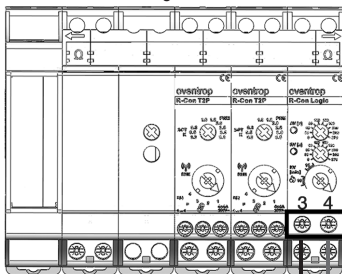
Abbildung 22: Verkabelung für Brenneranschluss an Logik-Modul
