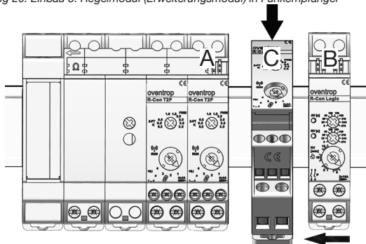
Abbildung 20: Einbau 3. Regelmodul (Erweiterungsmodul) in Funkempfänger
