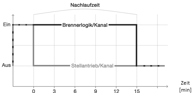
Abbildung 43: Diagramm Nachlaufzeit der Brennerlogik
