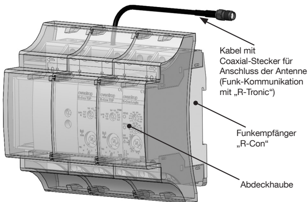
Abbildung 3: Frontansicht des Funkempfängers „R-Con“
