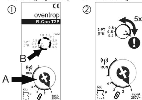
Abbildung 34: Zurücksetzung Regelmodul „T 2P“ auf Werkseinstellungen
