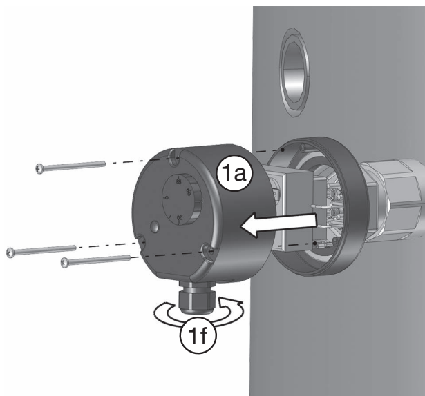
Abbildung 12: Innenansicht der Regler-/Begrenzer- kombination
