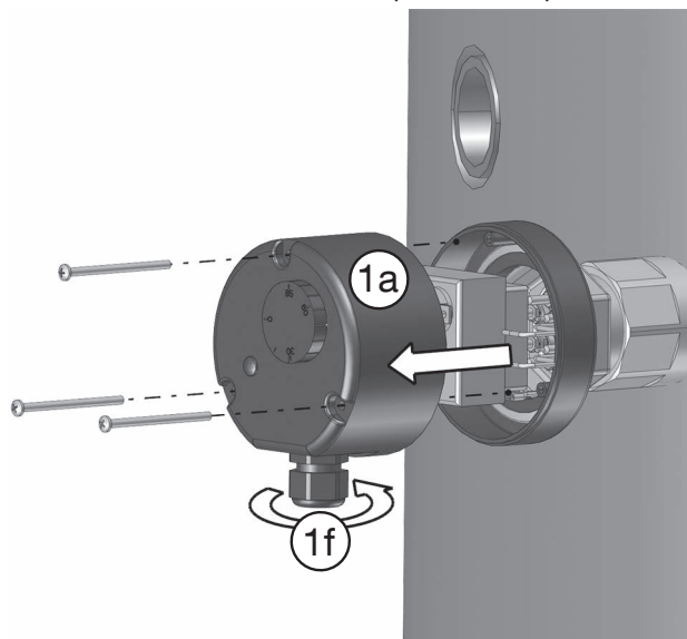
Figure 11: Démonter la cuvette supérieure, desserrer le presse-étoupe de câble
