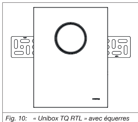
Fig. 10: « Unibox TQ RTL » avec équerres
