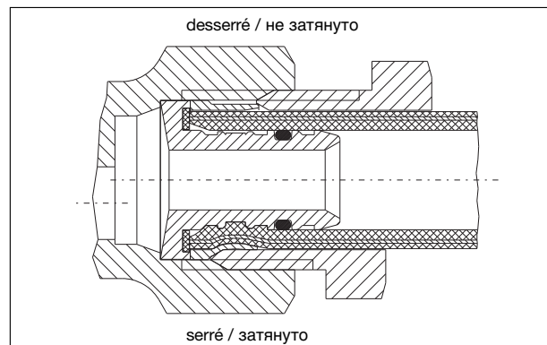
Ecrou et bague de serrage pour pièce à raccordement femelle Присоединение для внутренней резьбы
