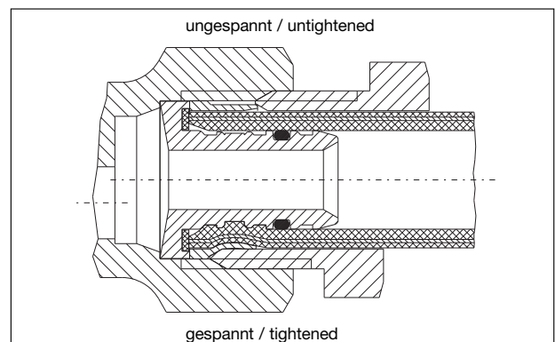
Klemmringverschraubung für Innengewindeanschluss Compression fittings for connections with female thread
