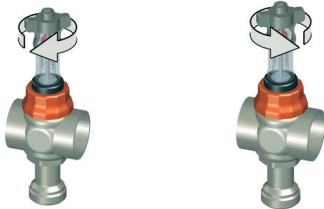
Fig. 7: Schließen und Öffnen der Einsätze
