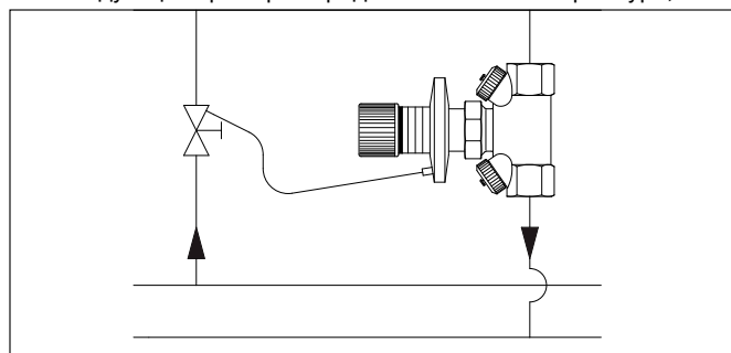
Пример: Регулирование перепада давления в системе с преднастраиваемыми термостатическими вентилями (стояки с небольшим и средним расходом).
