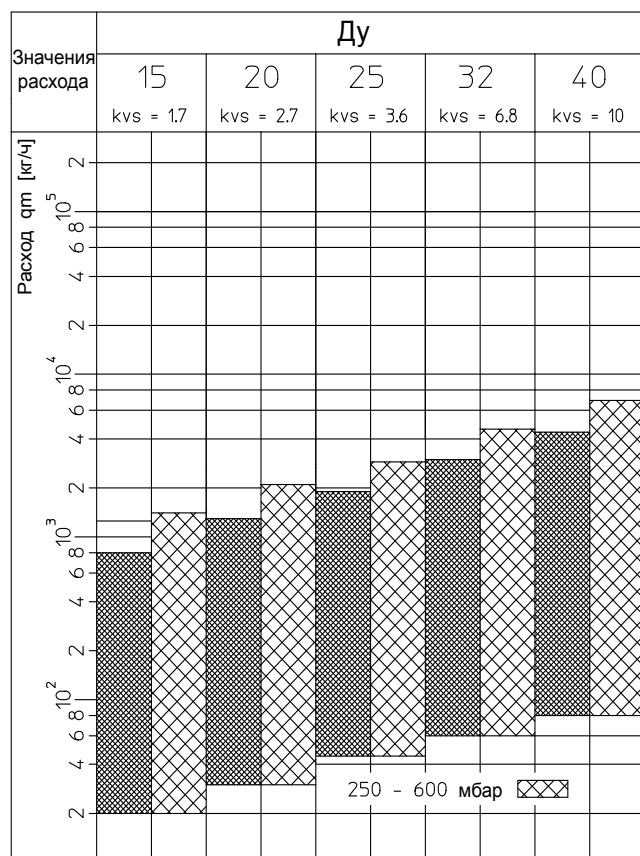
Значения расхода регулятора перепада давления „Нуссоп DTZ“ при перепаде давления в стояке 50–300 мбар или 250–600 мбар.
