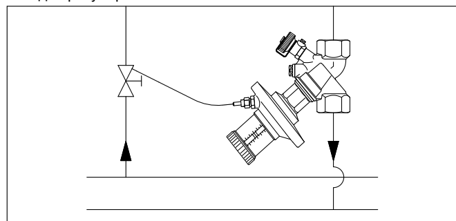
Пример: Регулирование перепада давления в системе с преднастраиваемыми термостатическими вентилями (стояки со средним и высоким расходом).
