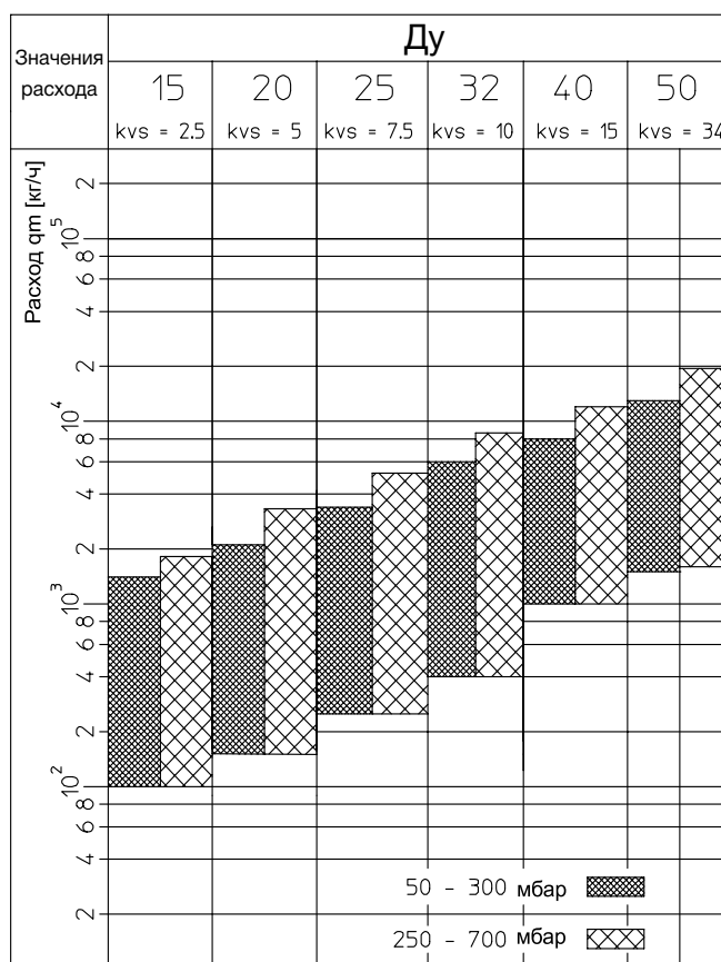
Значения расхода регулятора перепада давления „Нуссоп DTR“ при перепаде давления в стояке 50–300 мбар или 250–700 мбар.
