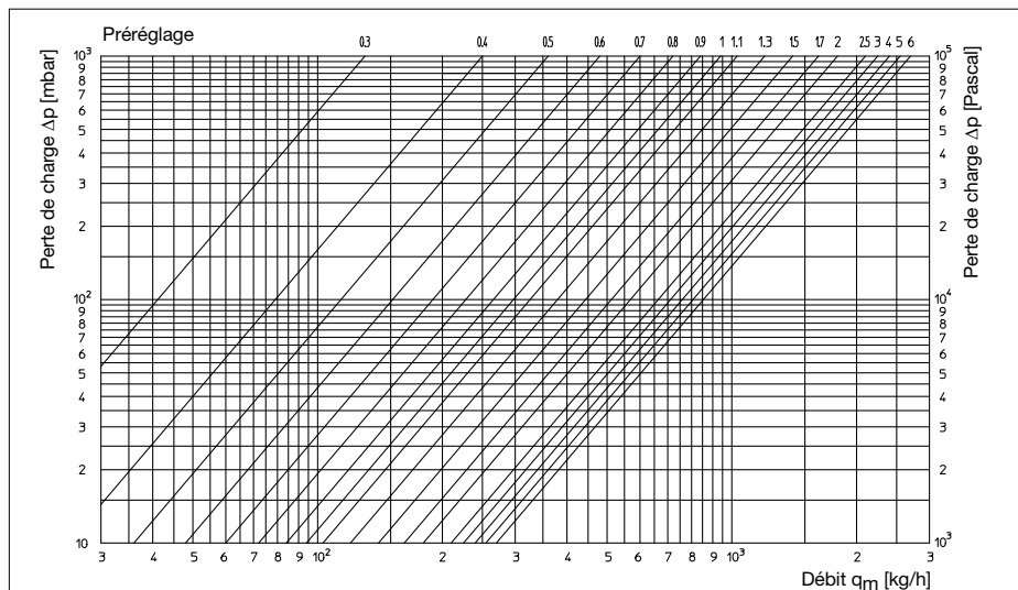
Fig. 9.1: Diagramme du robinet d'équilibrage «Hycococon VTZ» DN 20
