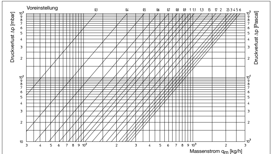
Abb. 9.1: Diagramm „Hycocn VTZ“ Strangregulventil DN 20
