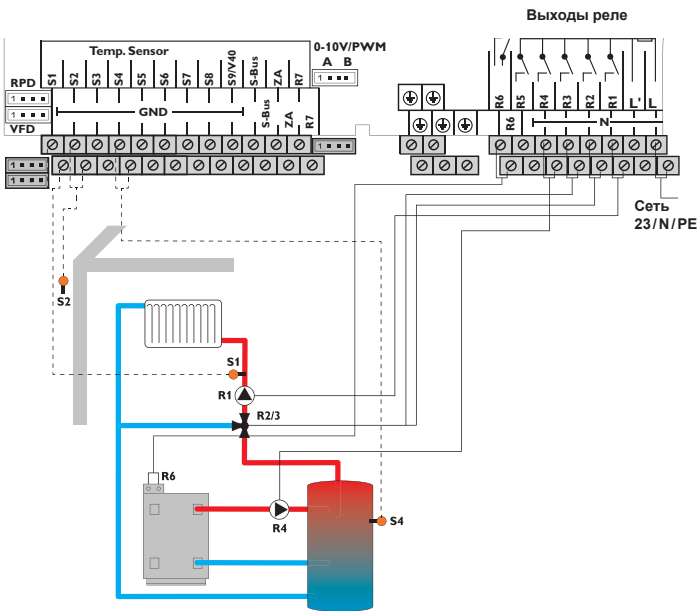
Схема 3: смешанный нагревательный контур с дополнительным нагревом (запрос и нагнетательный насос котла)
