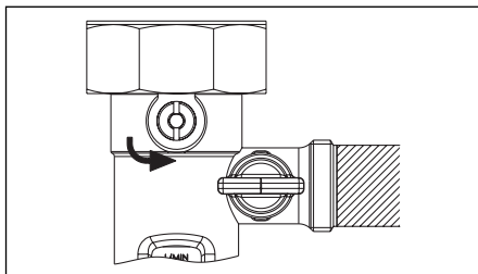
Abb. 6.20 Position Stellschraube
