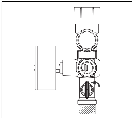
Abb. 6.17 Entleerungskugelhahn Sicherheitsgruppe
