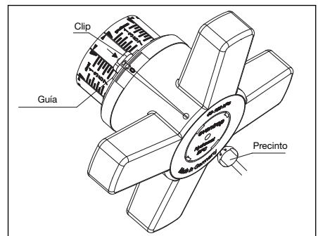
Fig. 7.2 Bloqueo del volante
