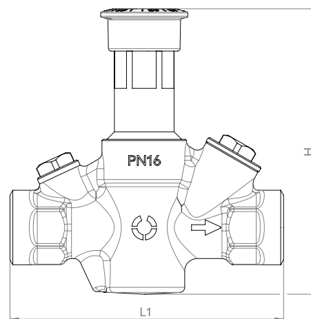
Fig. 2: Encombres latéraux
