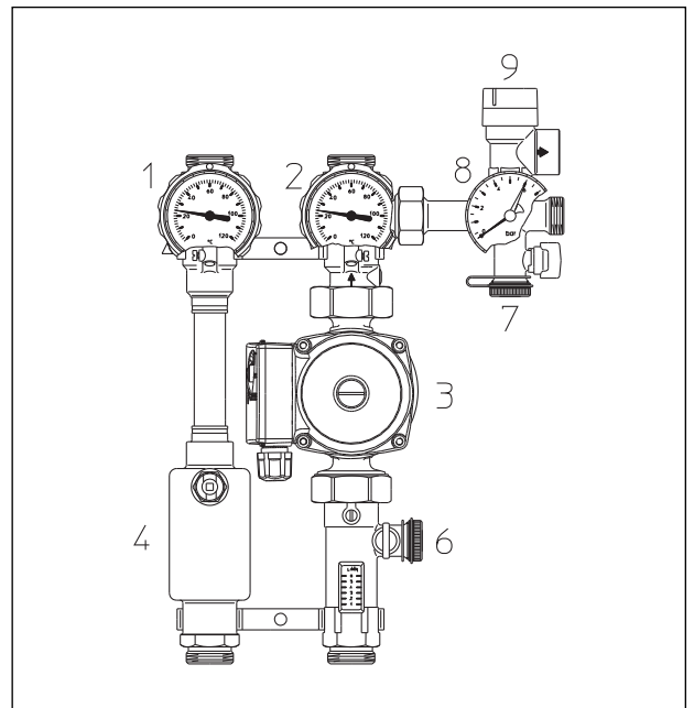
Fig. 23: Station solaire «Regusol L»
