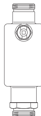
Fig. 4: Pot de purge, réf. OV 136 42 60
