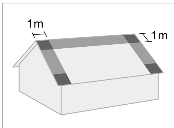
Bild 11: Mindestabstand des Kollektorfeldes vom Dachrand 1m. (Quelle: BDH, Informationsblatt Nr. 34, Ausgabe 04/2008)
