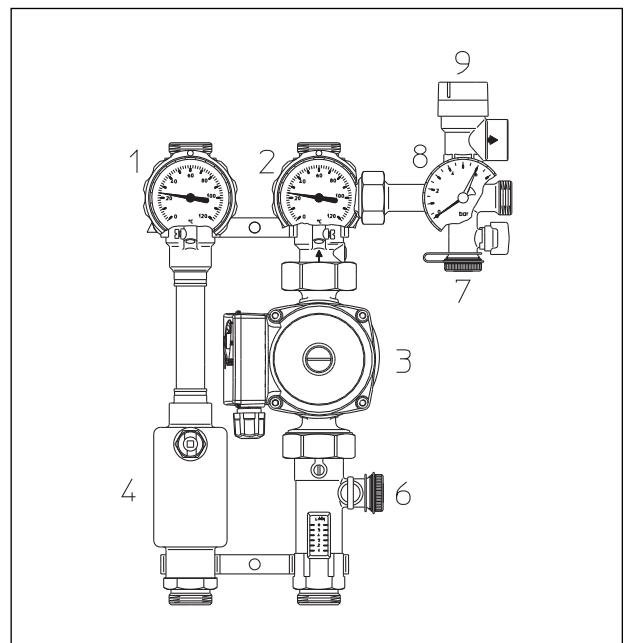
Bild 16: „Regusol L“-Solarstation
