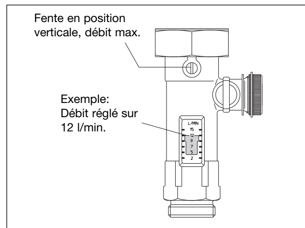
Fig. 26: Débitmètre avec vis de réglage
