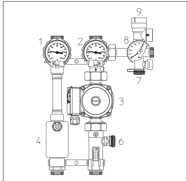
Bild 19: „Regusol L“-Solarstation
