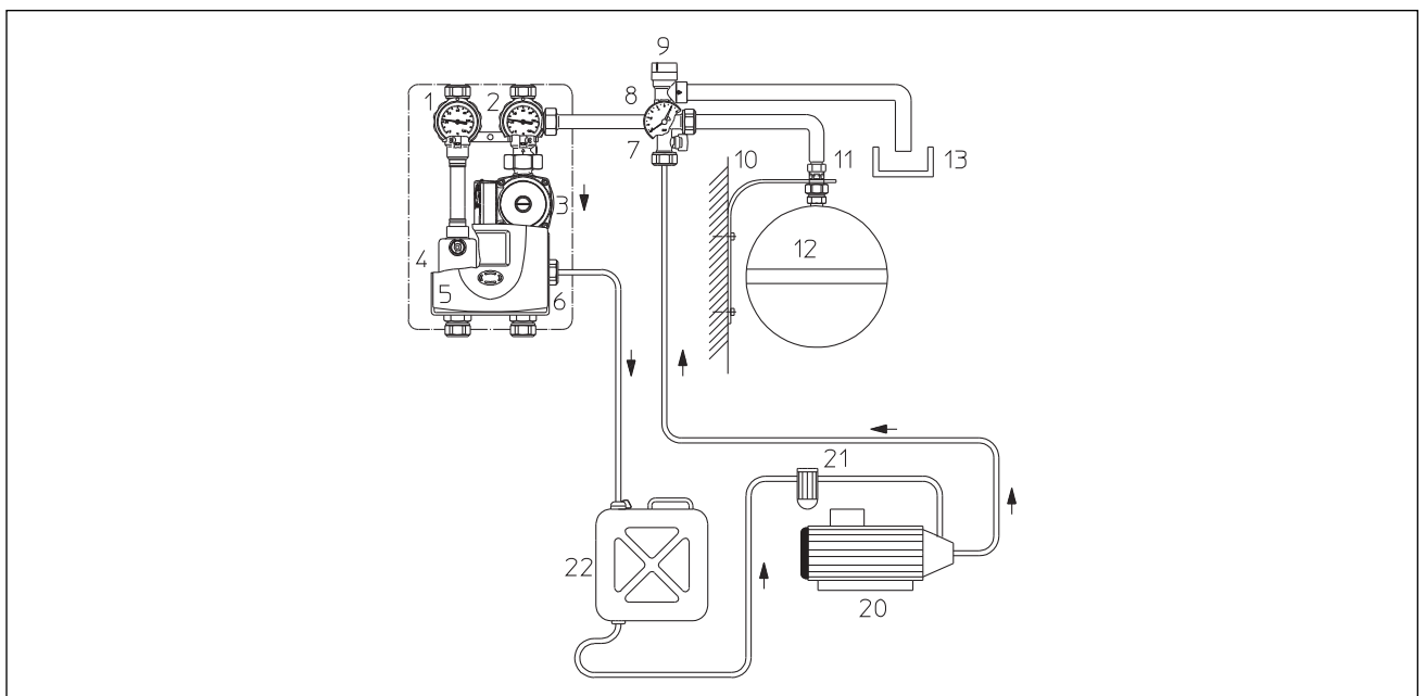
Bild 22: Pumpenstrang entlüften
