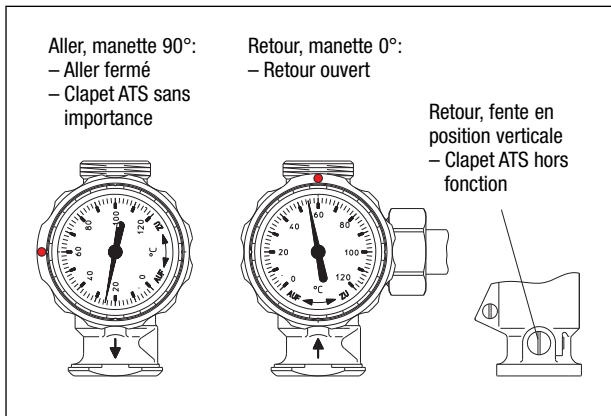
Fig. 21: Position des robinets à tournant sphérique
