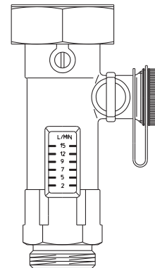
Bild 5: Durchflussmesser, OV Art.-Nr. 136 41 60/61/62
