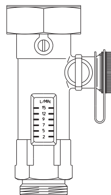
Fig. 5: Débitmètre, réf. OV 136 41 60/61/62
