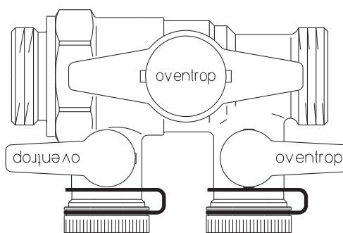
Fig. 6: Ensemble de remplissage et de rinçage, réf. OV 136 30 51
