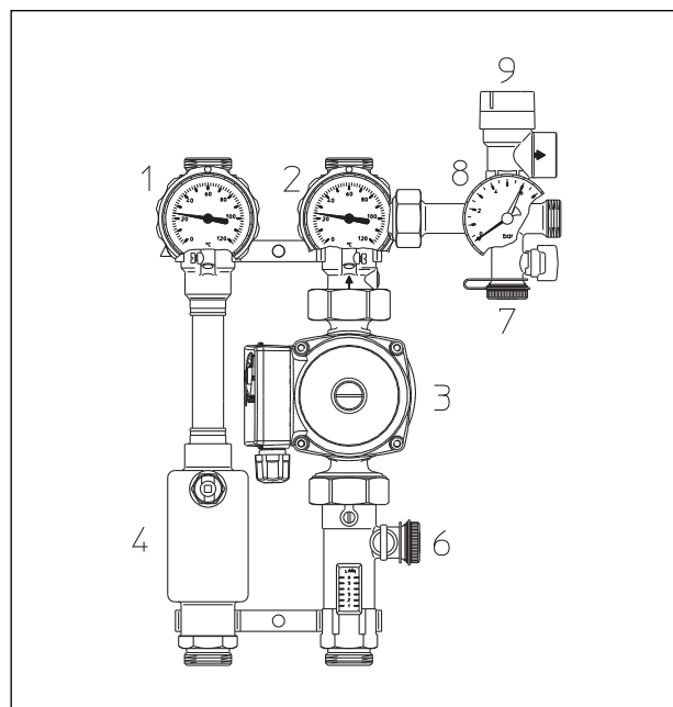
Bild 2: „Regusol L“-Solarstation
