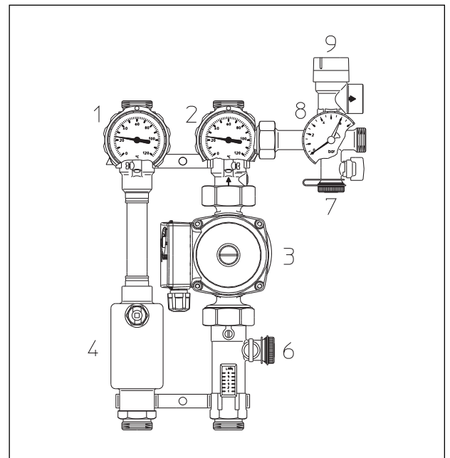
Bild 23: „Regusol L“-Solarstation
