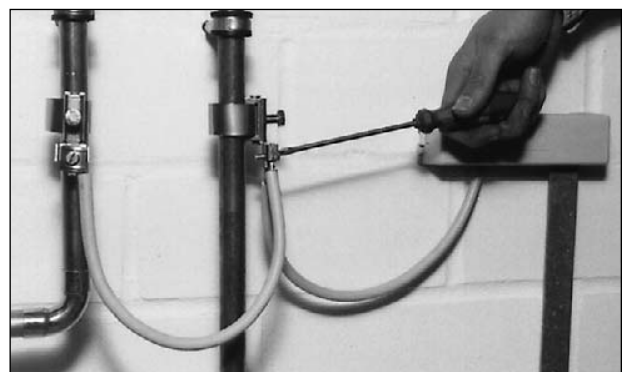
Bild 9: Für Potentialausgleich Erdungsschellen an beiden Solarkreisrohren anbringen und mind. 6 mm² Kabel mit Hauptpotentialausgleichsschiene verbinden.
