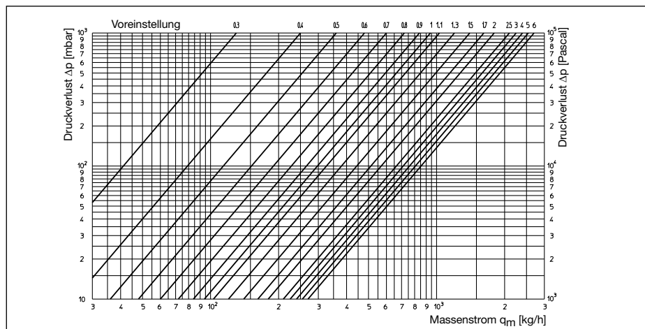
Diagramm 7.2: Druckverlust „Hycocn VTZ“ Strangreguliertventil DN 20
