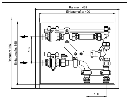
Abb. 3.1: Abmessungen seitliche Anbindung
