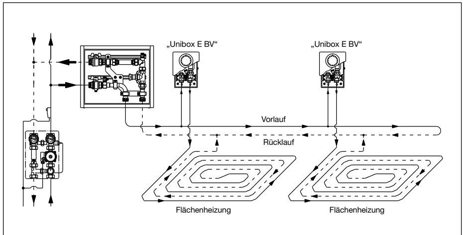
Abb. 5.2: Beispielskizze Anbindung seitlich
