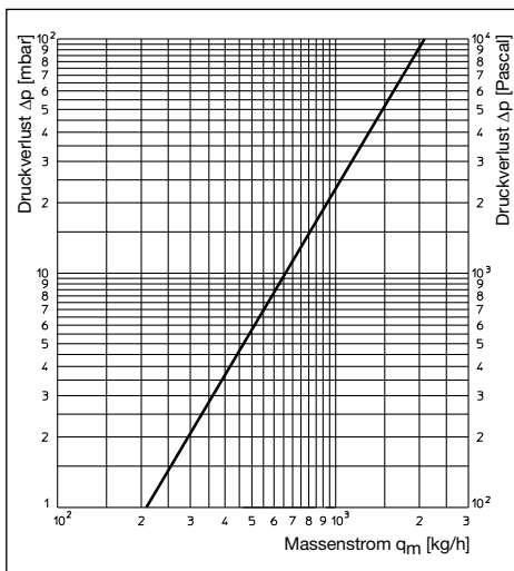
Abb. 7.1: Druckverlust „Floorbox“
