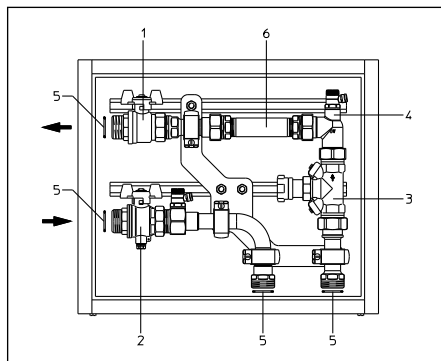
Abb. 4.1: Übersicht seitliche Anbindung
