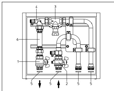
Abb. 4.2: Übersicht untere Anbindung
