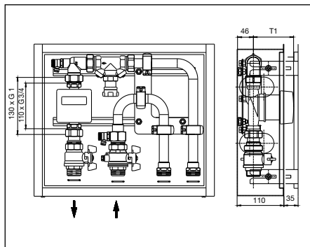
Abb. 5.1: Einbautiefe „Floorbox“
