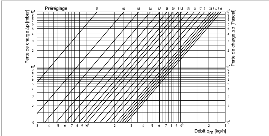
Illustr. 7.2: Perte de charge robinet d'équilibrage «Hyccon VTZ» DN 20
