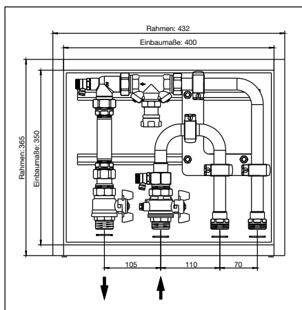
Abb. 3.2: Abmessungen untere Anbindung
