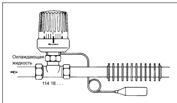
Двухтрубная система охлаждения
