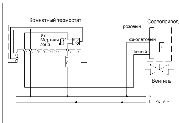
Схема переключения
