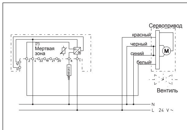
Схема переключения
