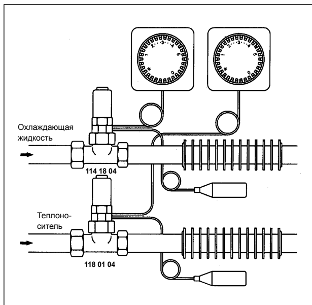
Четырехтрубная система с 2 теплообменниками
