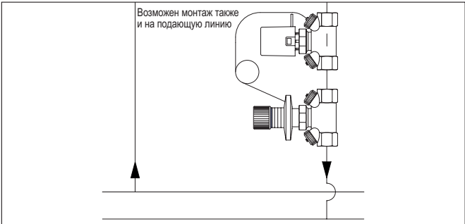
Пример: Регулирование расхода с помощью регулятора перепада давления „Hysocoon DP“ и регулирующего вентиля „Hysocoon TM“.
