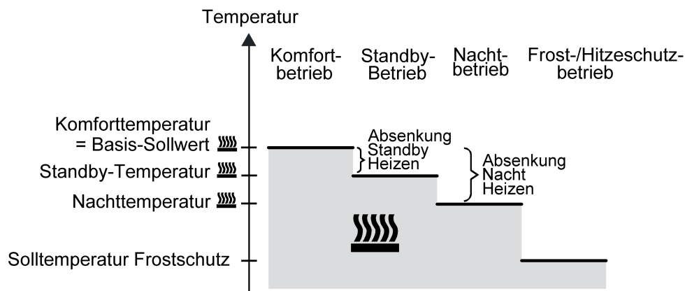
Bild 32: Solltemperaturen in der Betriebsart "Heizen"
