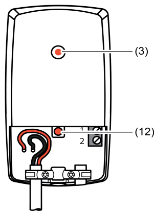
Bild 8: Programmier- und -LED
