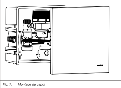
Fig. 7: Montage du capot
