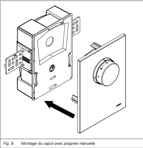
Fig. 9: Montage du capot avec poignée manuelle
