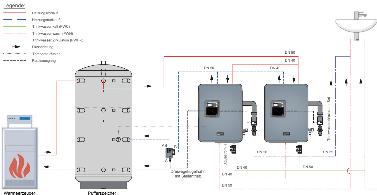
Abb. 3.6: Anlagenschema mit zwei Frischwasser-Stationen „Regumaq X-80“ („Tichelmann-System“)
