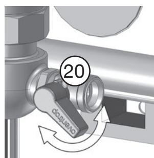
Abb. 5.10: Speicherkreisseite entlüften
