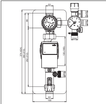
Abb. 4.1 Pumpenstrang „Regusol PH-130 (180)“ DN 25
