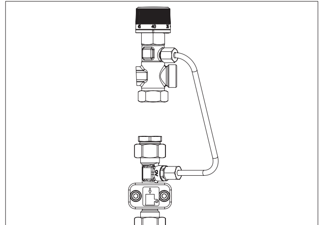
Abb. 5: Einbau Kupferrohr Regudis W-HTU/TU und Regudis W-HTF
