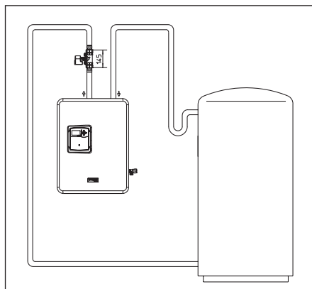
Fig. 5.1 Montage dans une station «Regumaq X-80»
