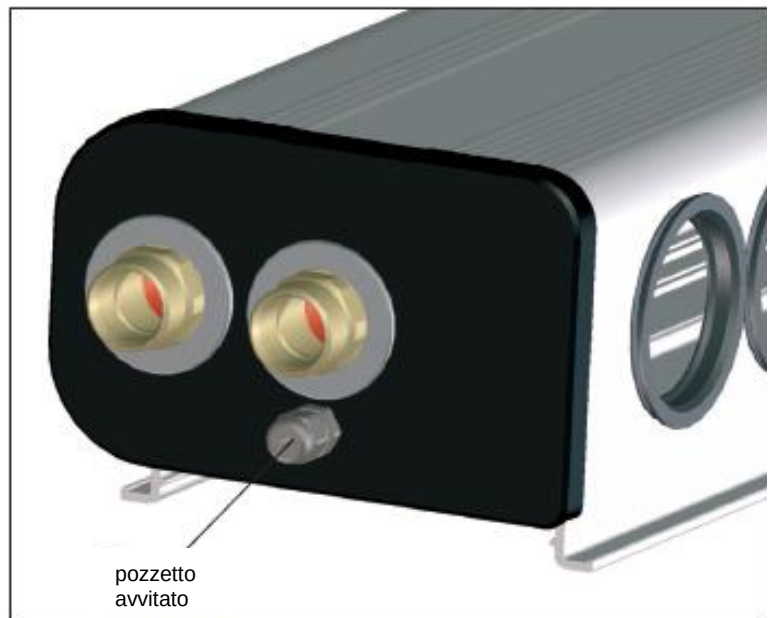
Illustr. 28: Copertura a tappo di sinistra con pozzetto avvitato per il fissaggio di un sensore di temperatura (es. PT1000)
