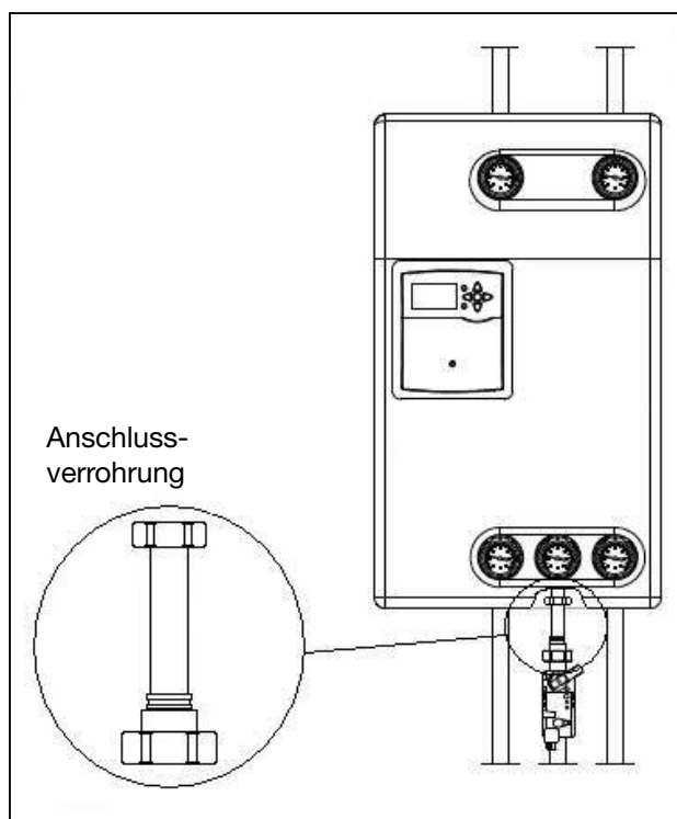
Anschlussverrohrung 1389082 Einbaubeispiel
