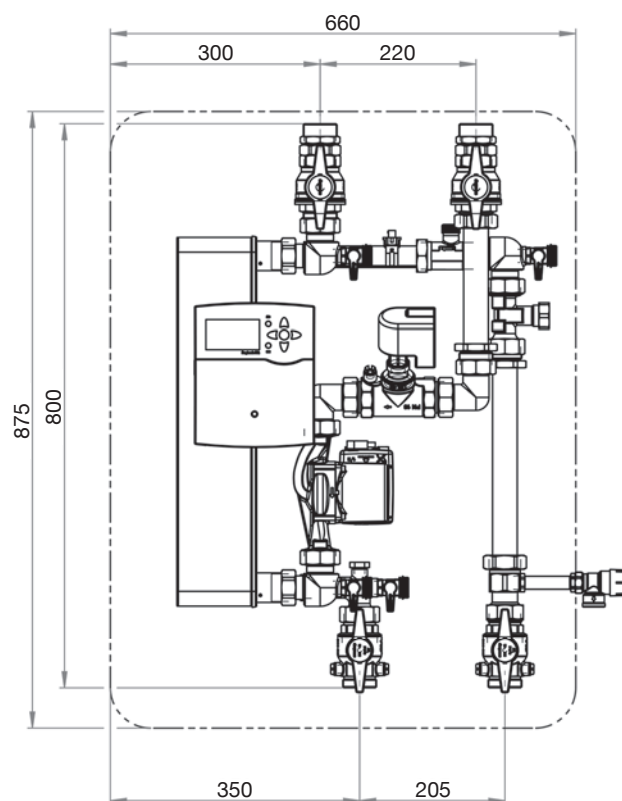
Fig. 3.8: Encombremments «Regumaq X-80» (vue avant)
