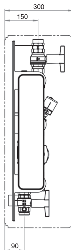
Fig. 3.9: Encombremments «Regumaq X-80» (vue de côté)
