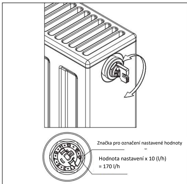
Obr. 4: Nastavení průtoku
