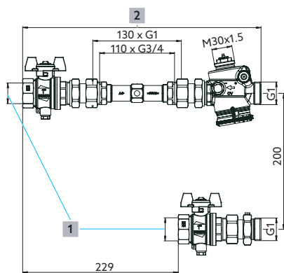
Abb. 4: Abmessungen Durchgangsausführung
