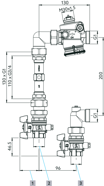
Fig. 3: Encombrenements du modèle équerre
