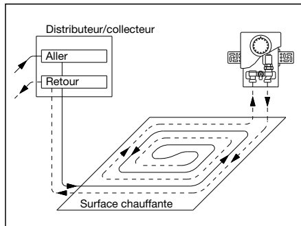
Croquis d'installation
