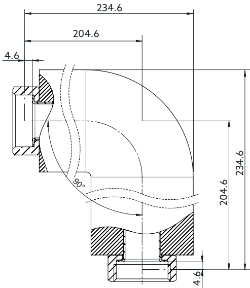
Abb. 5: Abmessungen Rohrwinkelstück
