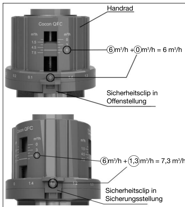
Abb. 3 Einstellbeispiele
