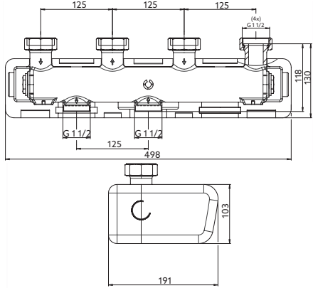
Fig. 2: Dimensions
