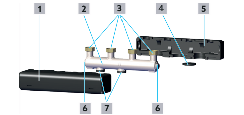
Abb. 1: Aufbau
