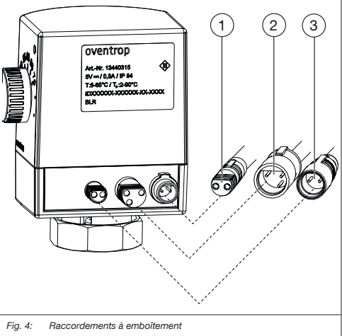
Fig. 4: Raccordements à emboîtement
