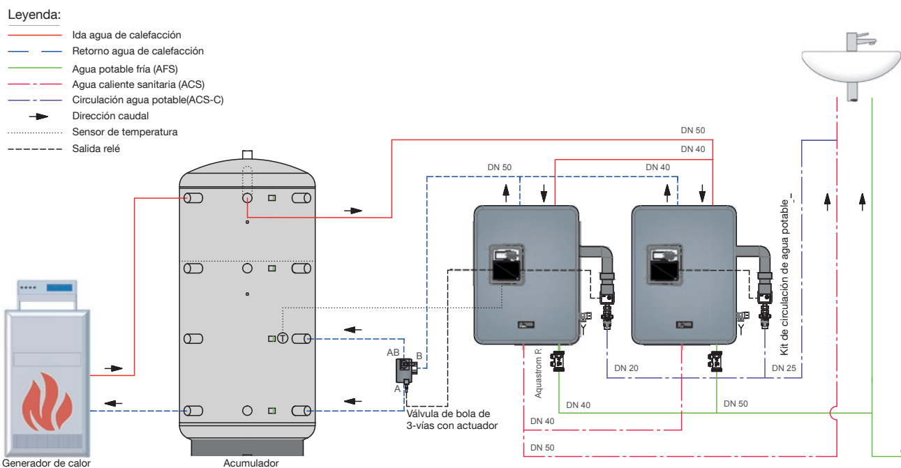
fig. 3.6: Diagrama de sistema con dos estaciones de agua potable “Regumaq X-80” (sistema “Tichelmann”)
