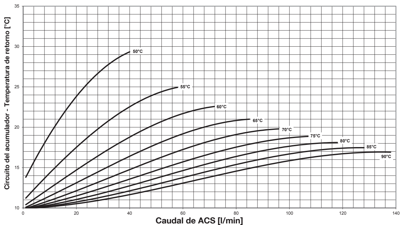
Temperatura de retorno del circuito del acumulador a diferentes temperaturas de caudal - Calentamiento de agua potable de 10°C a 50°C -
