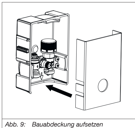
Abb. 9: Bauabdeckung aufsetzen
